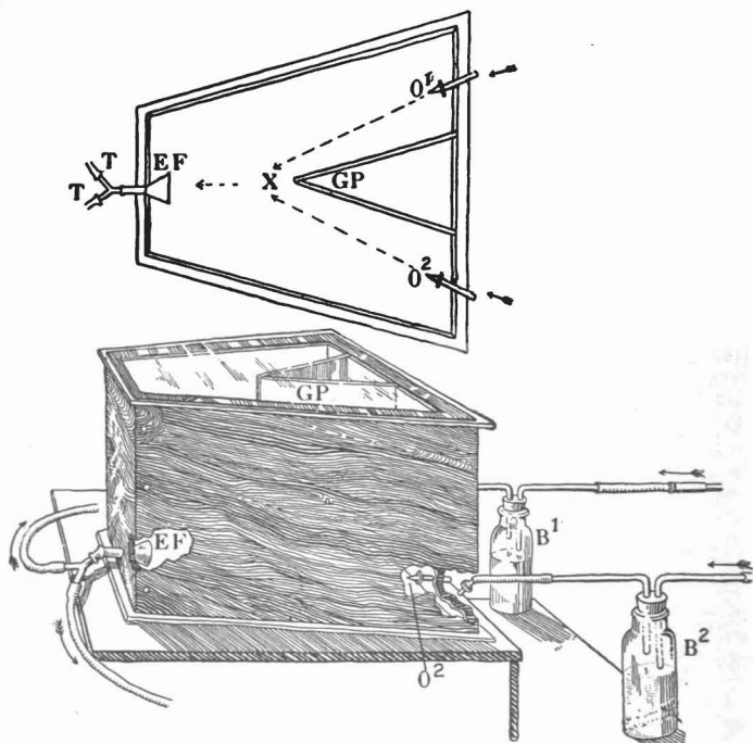
FIG. 14. OLFACTORY APPARATUS
